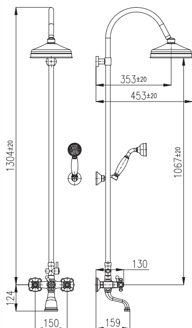
KS0020 metal / метал.
