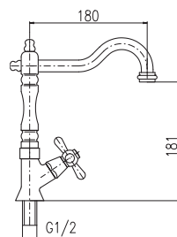
MK194/8 MK594/8 Chrome – Хром
