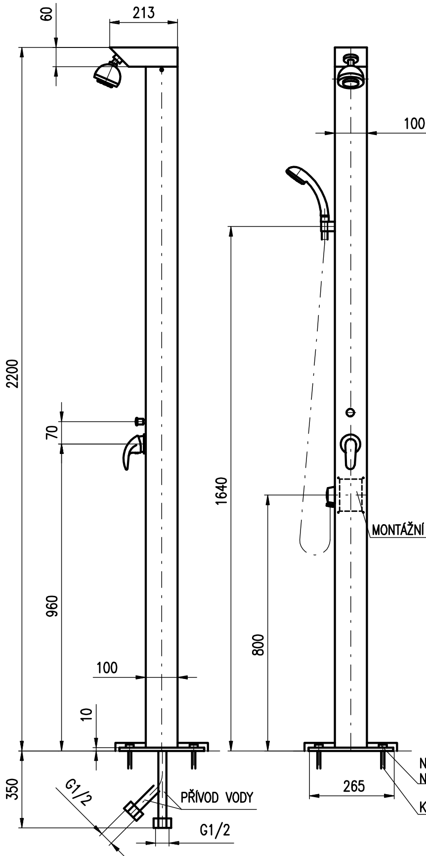
Z1220 – montážní otvor
